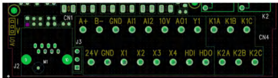
图 2-3 (非隔离版本) 控制回路端子布置图
