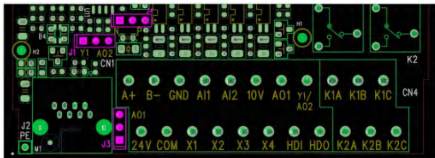
图 2-4 (隔离版本) 控制回路端子布置图
