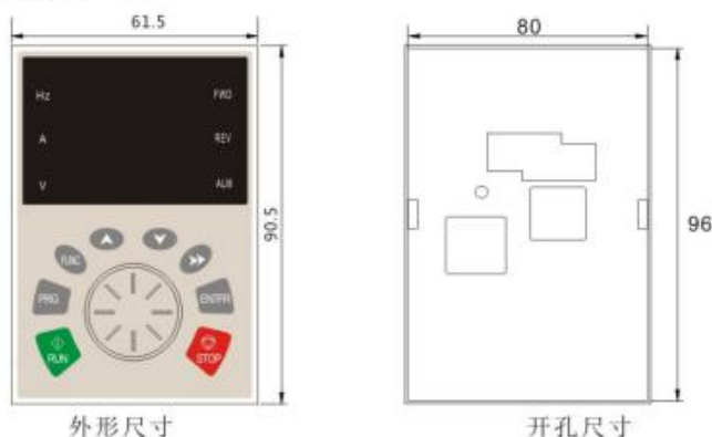
图1-4外引键盘的外型尺寸
